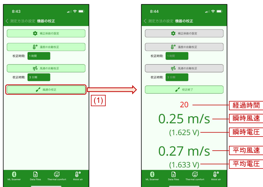
Fig. 3.12 手動風速校正
