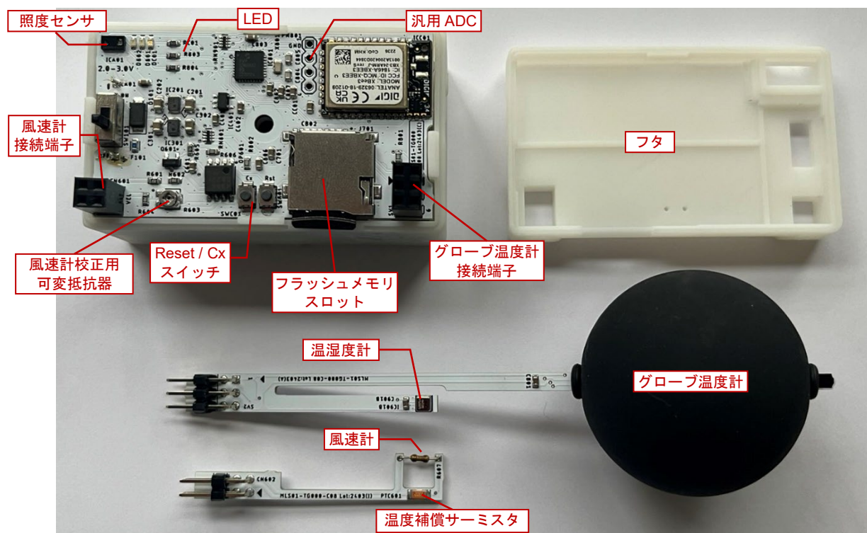
Fig. 2.4 子機（M-Logger）の要素
